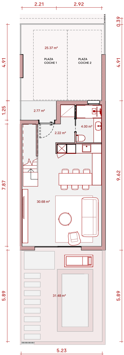
Planta Baja
