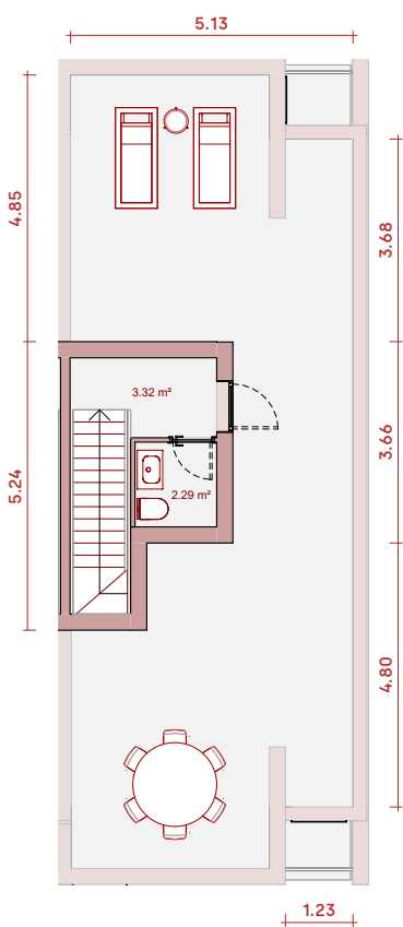
Planta Cubierta
