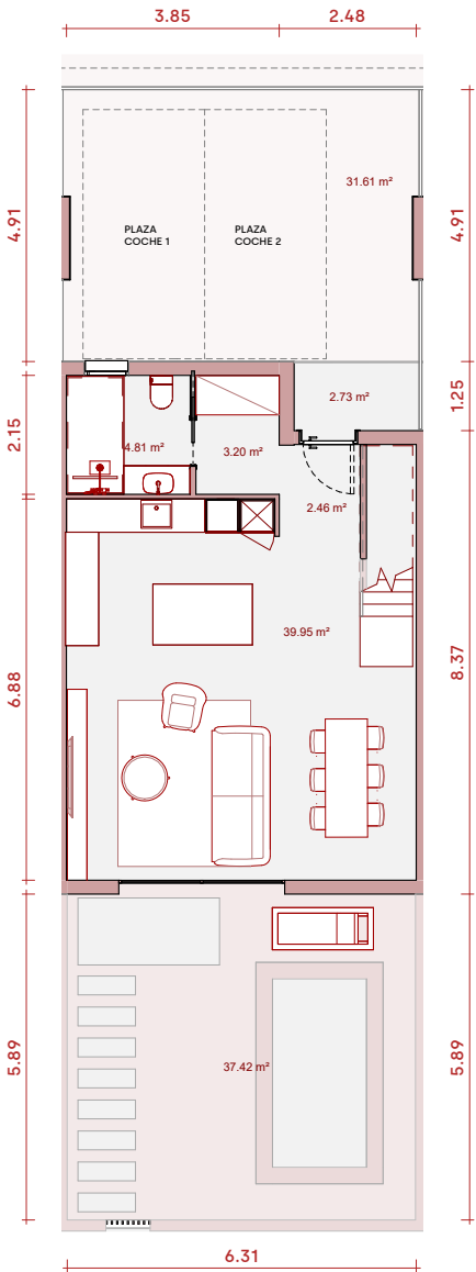
Planta Baja
