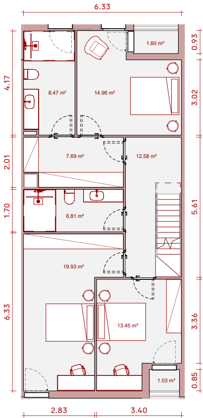
Planta Primera
