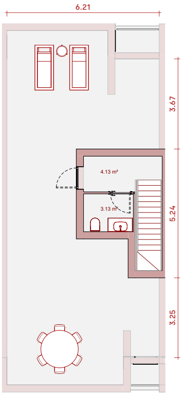
Planta Cubierta
