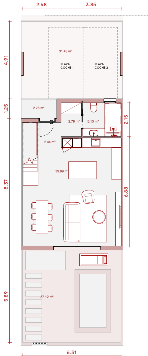
Planta Baja
